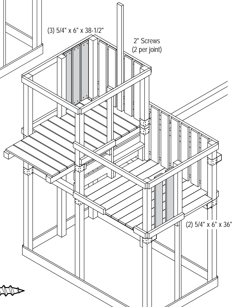
Fig. 25a
