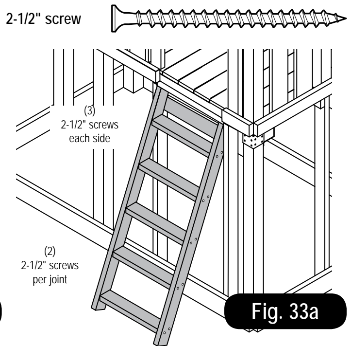
Fig. 33
