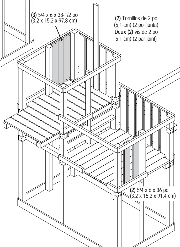
Fig. 25a
