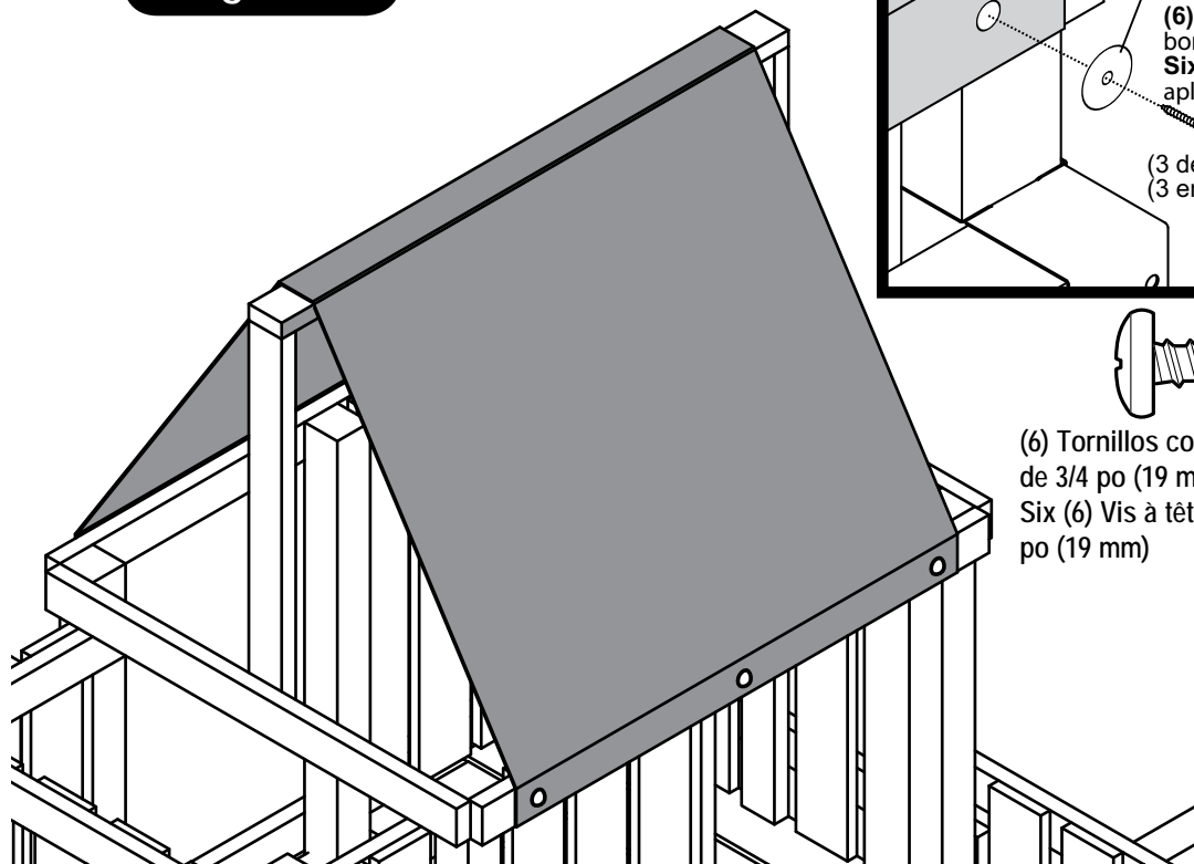
Fig. 34a
